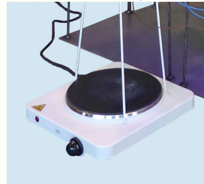
5 Vandet lander på den varme kogeplade og fordamper
